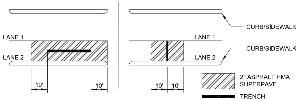
FIGURE 1 LONGITUDINAL TRENCH
